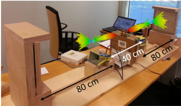
Fig. 14. Chipless RFID tags and UWB RA antenna testbed.
